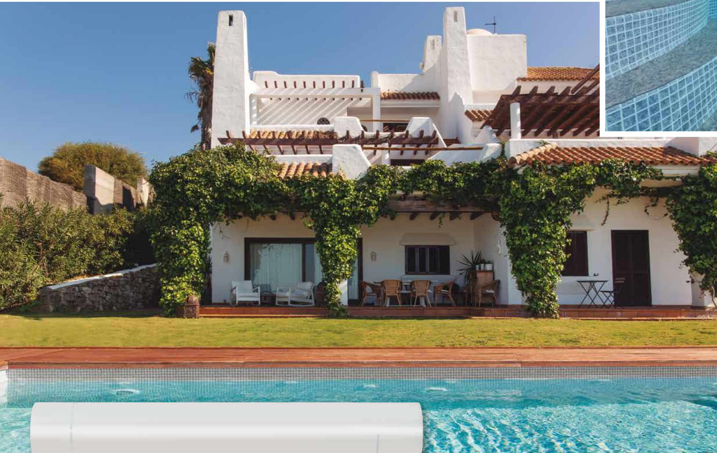
Etna RENOLIT ALKORPLAN CERAMICS Breite Dicke Art. Nr. Etna 1,65 m 2 mm 35617204
